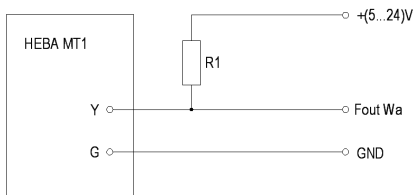
Рисунок 2.1 Подключение импульсных выходов
