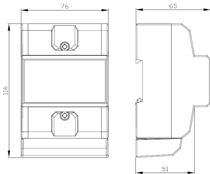
Внешний вид счётчиков НЕВА МТ 12Х
