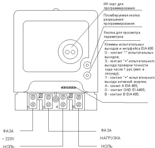
Схема подключения счётчиков НЕВА МТ 11Х
