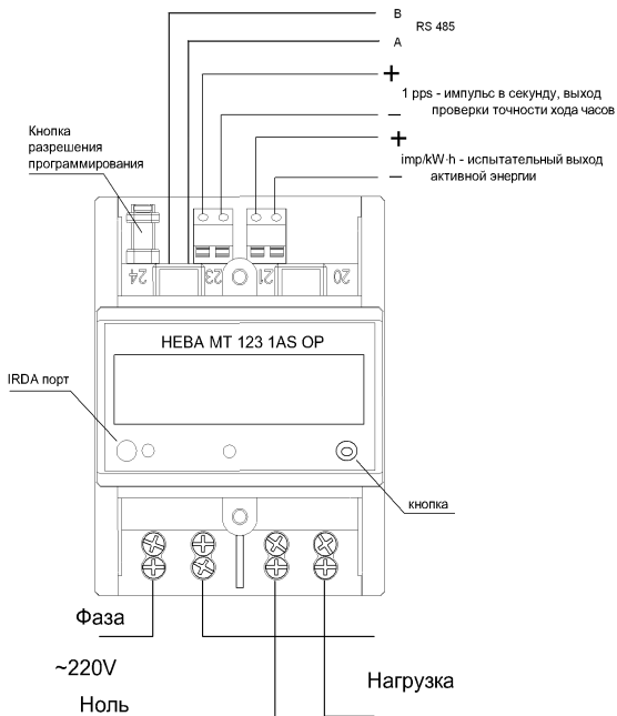
Схема подключения счётчиков HEBA MT 12X
